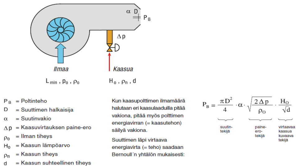
Kuva 1 Kaasupolttimen toimintaperiaate [1]
