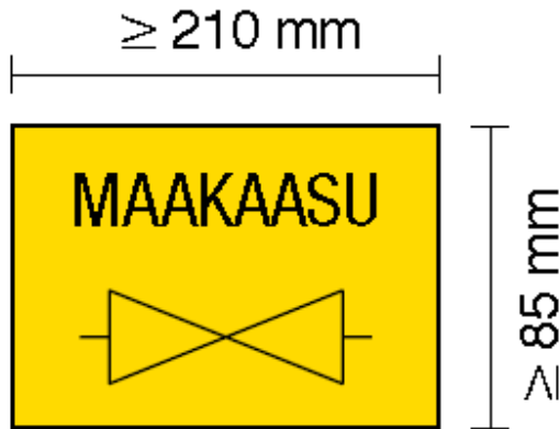
Kuva 5 Venttiilin tunnuskilpi.[1]
