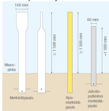
Kuva 3 Merkintäpaalu
